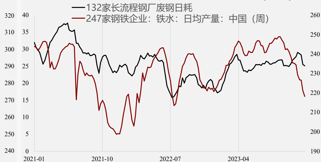
长流程废钢日耗和日均铁水产量对比(万吨)
