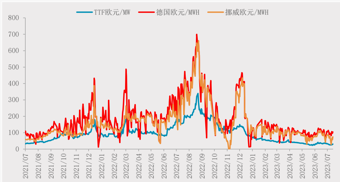
2.7 欧洲电价
