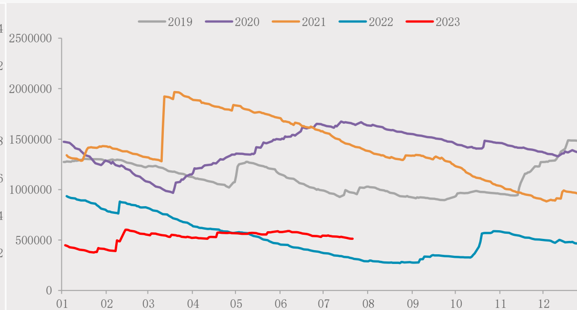
5.3LME库存
