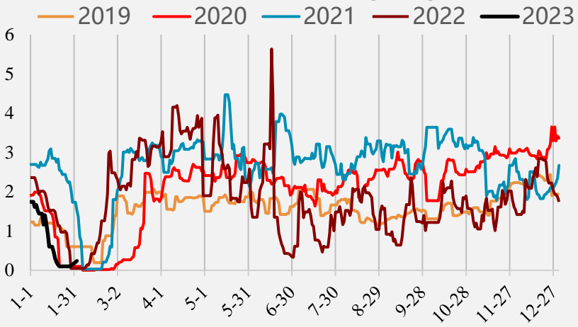
西南废钢到货量(万吨)
