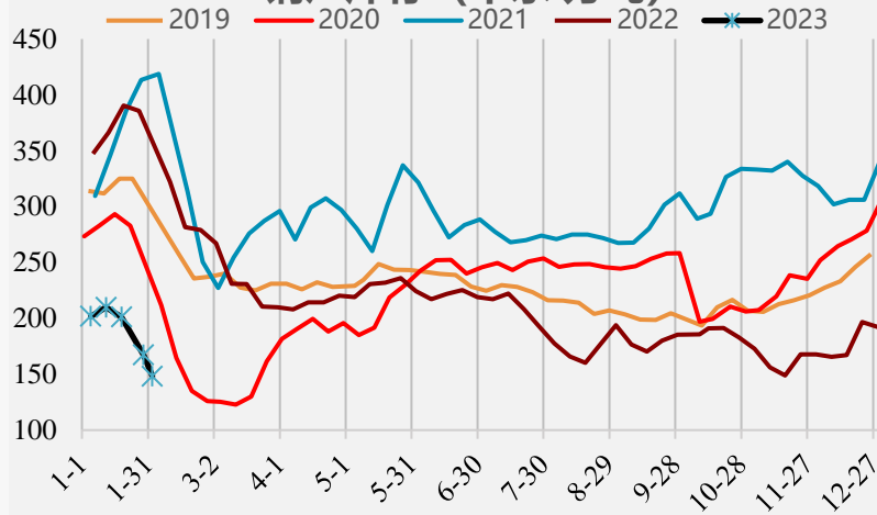
钢厂库存 (华东 万吨)
