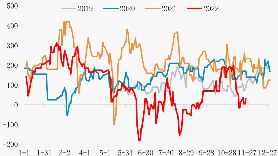
钢板料价差：张家港8mm-广州6mm
