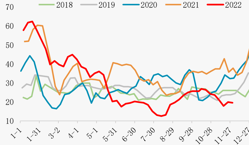
钢厂废钢库存(华中 万吨)
