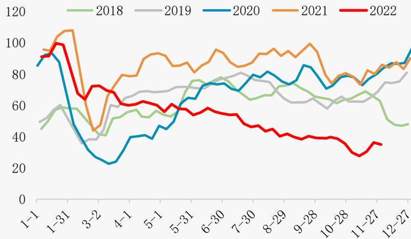
钢厂废钢库存(华北 万吨)
